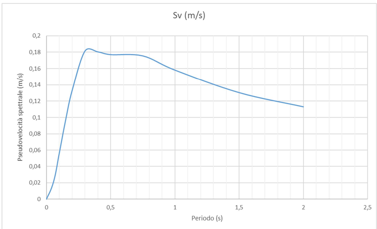
Fig. 9.2 – Spettro di risposta elastico in velocità su suolo rigido (475Y)
