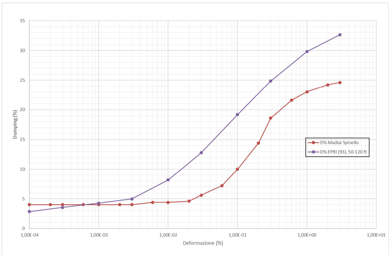
Fig. 9.5 – Curve di smorzamento
