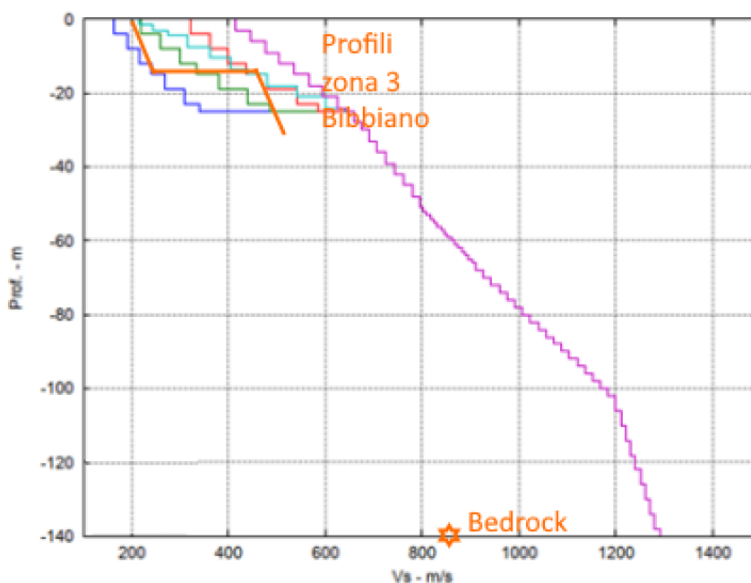
Fig. 31 - Confronto tra i profili di Vs misurati nella zona 3 con quelli medi utilizzati per il calcolo dei fattori di amplificazione riportati negli abachi per Ambiente di Appennino in caso di substrato non rigido a -25 m da p.c.
