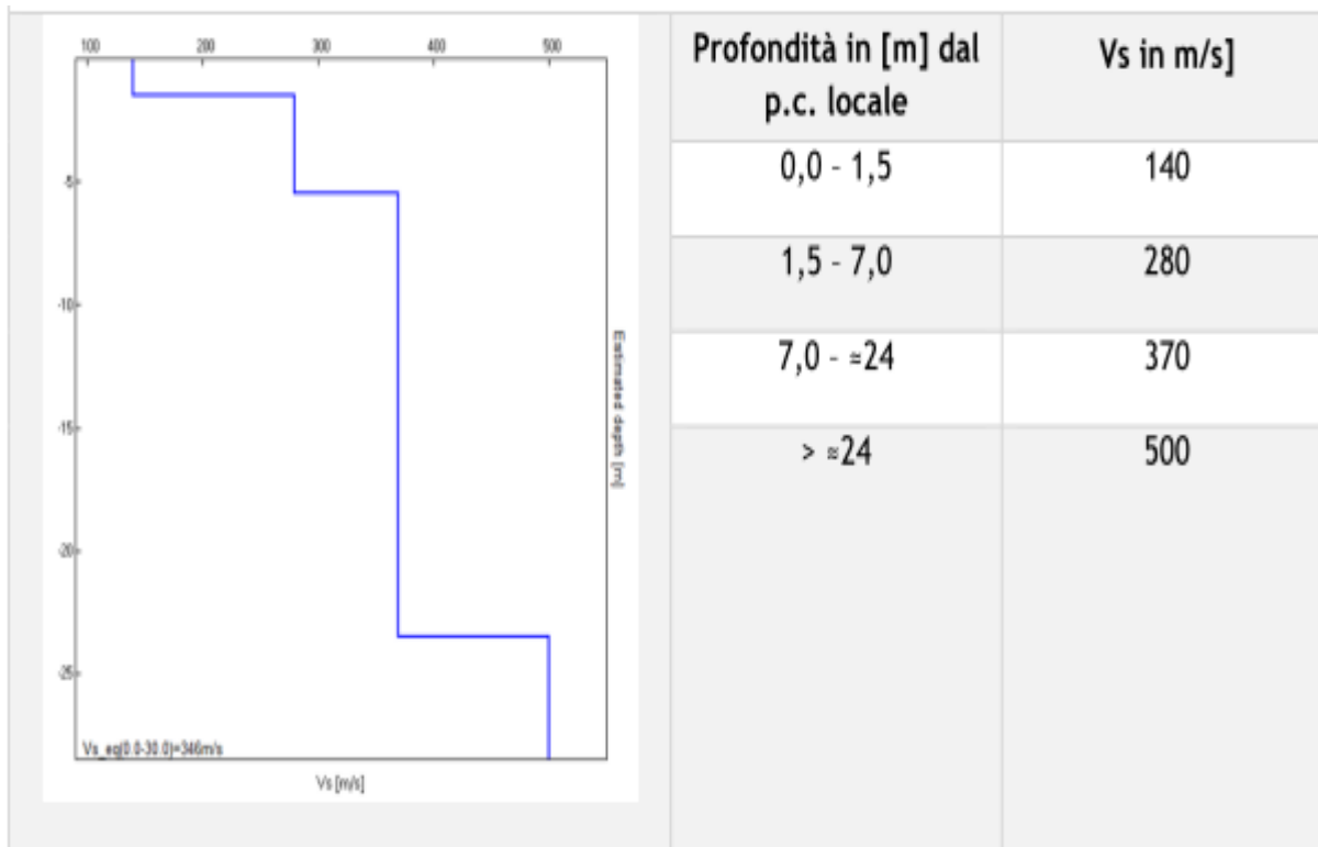
Fig. 13 - Profilo delle velocità delle onde S da prova MASW
