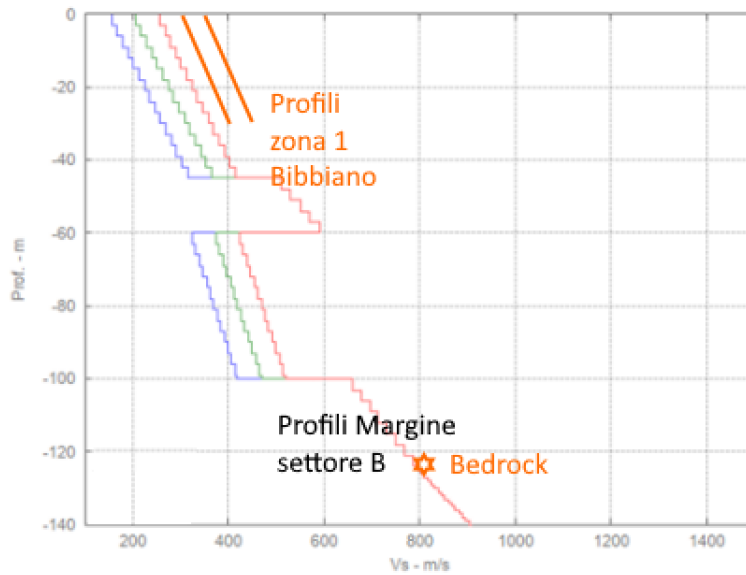
Fig. 26 - Confronto tra i profili di Vs misurati nella zona 1 con quelli medi utilizzati per il calcolo dei fattori di amplificazione riportati negli abachi per Ambiente di Margine di tipo B
