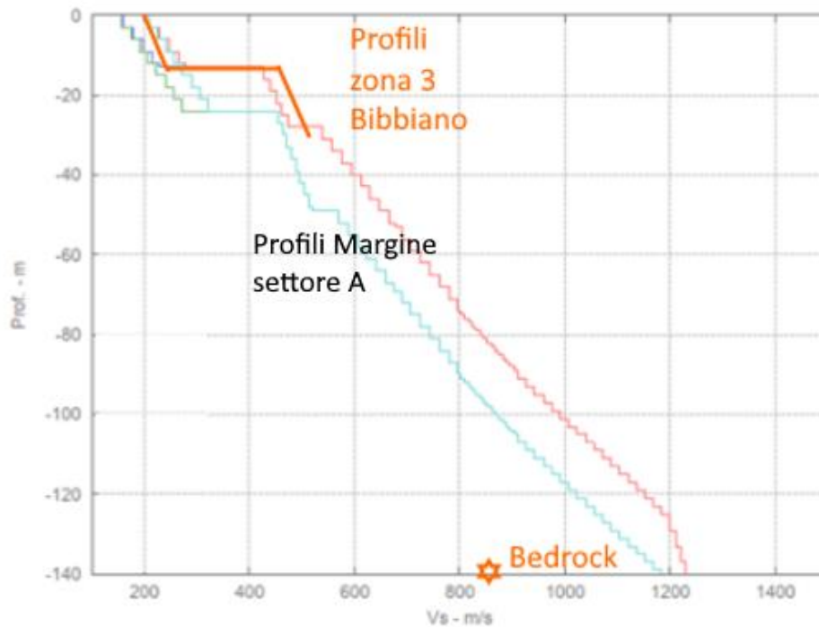
Fig. 29 - Confronto tra i profili di Vs misurati nella zona 3 con quelli medi utilizzati per il calcolo dei fattori di amplificazione riportati negli abachi per Ambiente di Margine di tipo A
