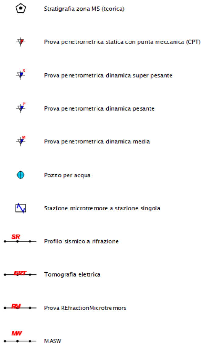
Fig. 21 – Legenda delle Carte delle indagini
