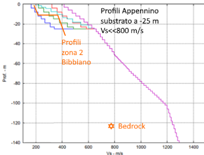
Fig. 30 - Confronto tra i profili di Vs misurati nella zona 2 con quelli medi utilizzati per il calcolo dei fattori di amplificazione riportati negli abachi per Ambiente di Appennino in caso di substrato non rigido a -25 m da p.c.
