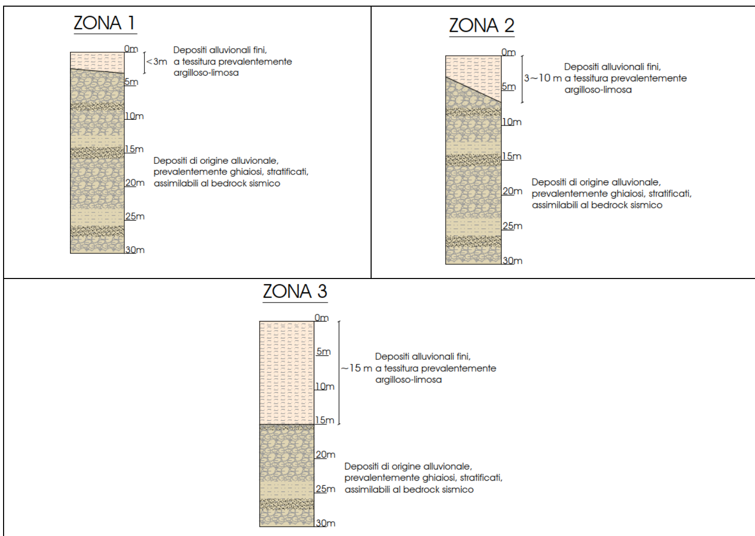
Fig. 25 - Colonne litostratigrafiche sintetiche, rappresentative delle microzone stabili suscettibili di amplificazioni locali
