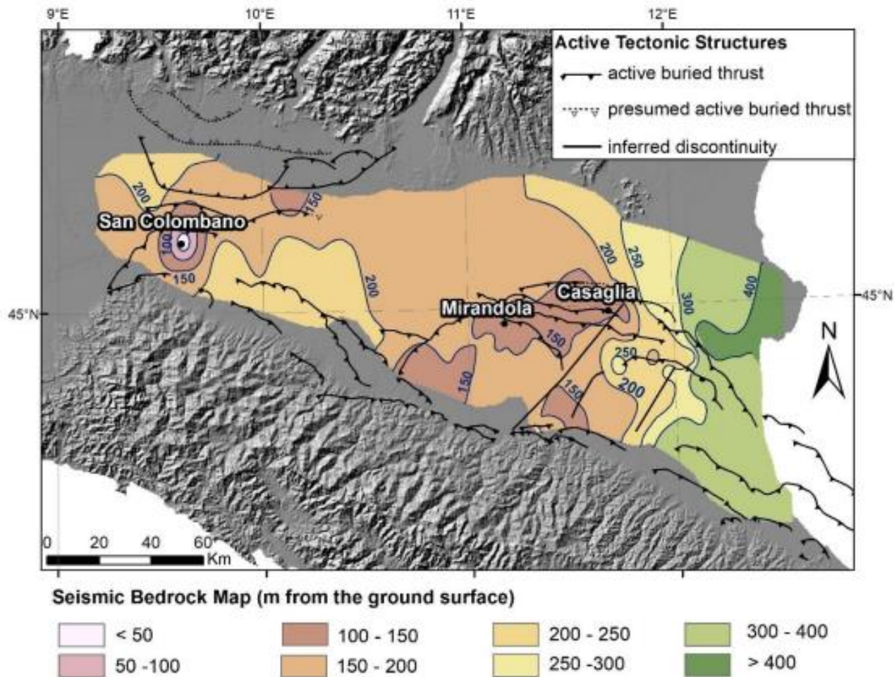
Fig. 20 - Mappa della profondità del bedrock sismico (da Mascandola et al., 2018)
