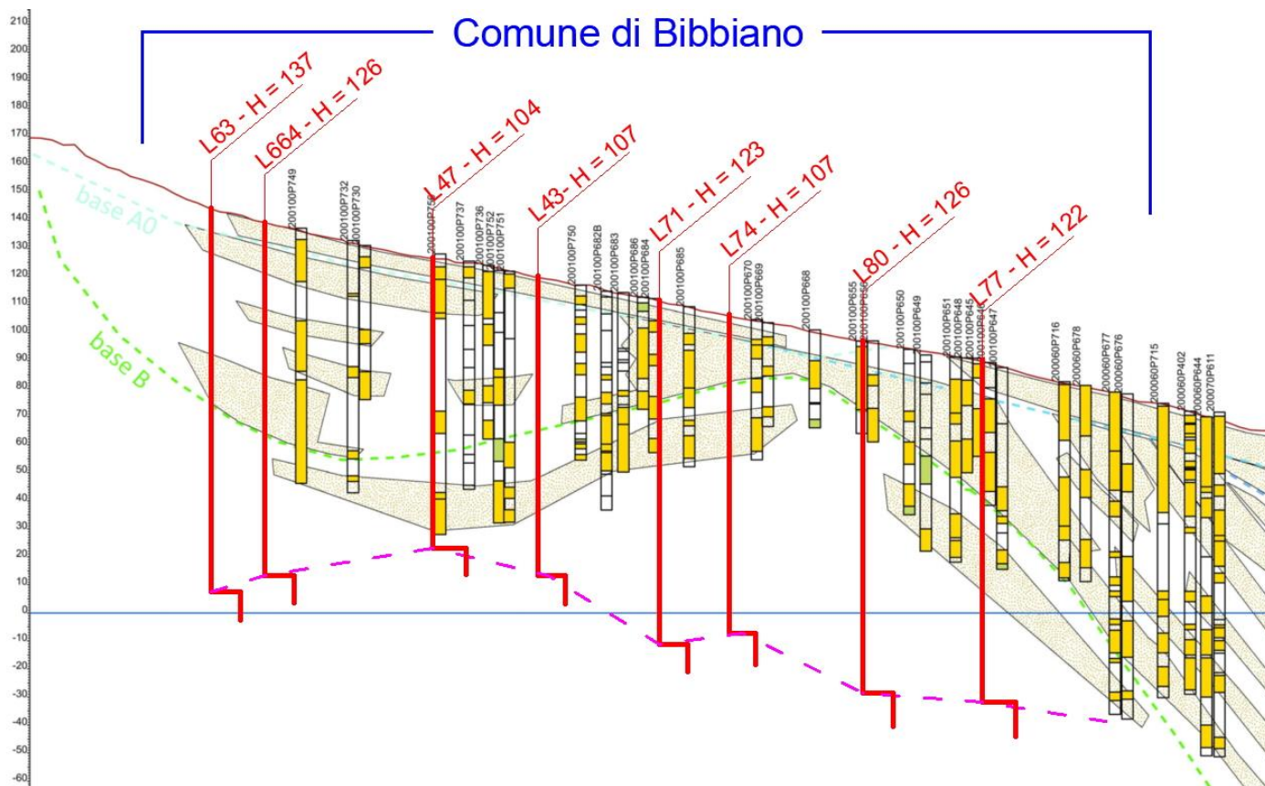
Fig. 19 - Stralcio della Sezione 6 tratta dal sito web del Servizio Geologico della Regione Emilia-Romagna con rappresentazione della superficie d'impedenza desunta dalle elaborazioni congiunte REMI-HVSR effettuate all'interno del presente studio
