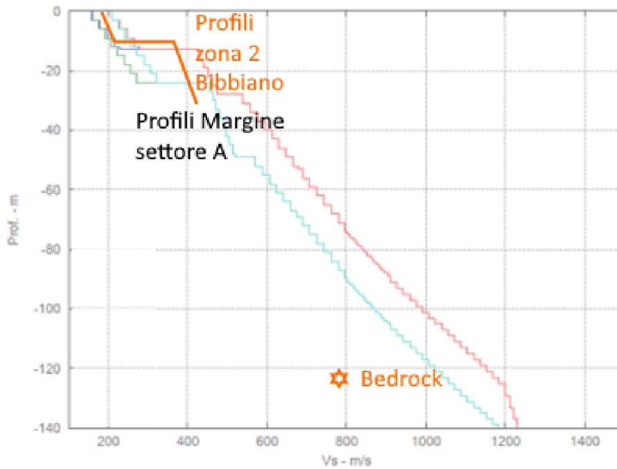
Fig. 28 - Confronto tra i profili di Vs misurati nella zona 2 con quelli medi utilizzati per il calcolo dei fattori di amplificazione riportati negli abachi per Ambiente di Margine di tipo A
