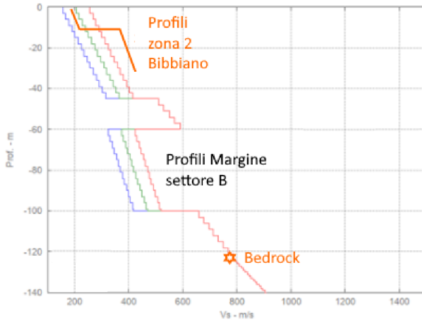
Fig. 32 - Confronto tra i profili di Vs misurati nella zona 2 con quelli medi utilizzati per il calcolo dei fattori di amplificazione riportati negli abachi per Ambiente di Margine di tipo B
