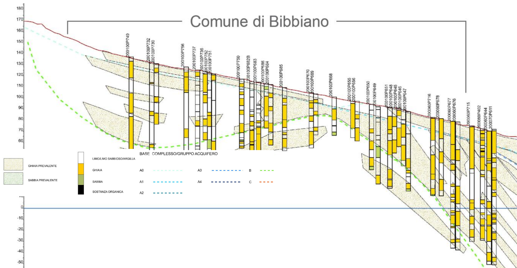
Fig. 23 - Stralcio della Sezione 135 tratta dal sito web del Servizio Geologico della Regione Emilia-Romagna
