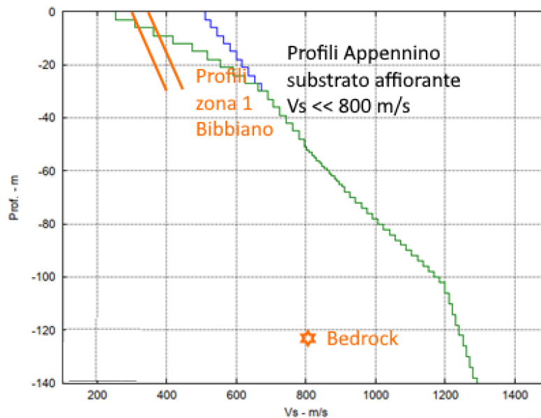
Fig. 27 - Confronto tra i profili di Vs misurati nella zona 1 con quelli medi utilizzati per il calcolo dei fattori di amplificazione riportati negli abachi per Ambiente di Appennino in caso di substrato non rigido affiorante o subaffiorante
