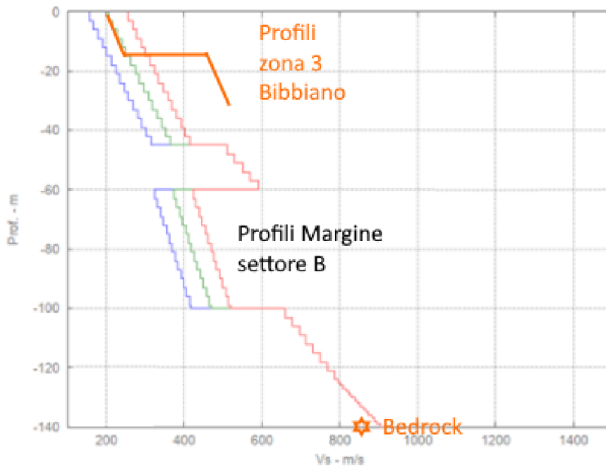
Fig. 33 - Confronto tra i profili di Vs misurati nella zona 3 con quelli medi utilizzati per il calcolo dei fattori di amplificazione riportati negli abachi per Ambiente di Margine di tipo B
