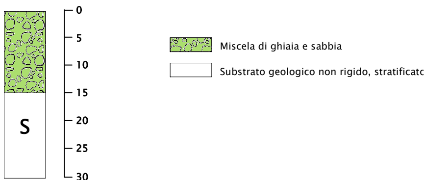
Figura 37 – Successione stratigrafica cod. 2003.
