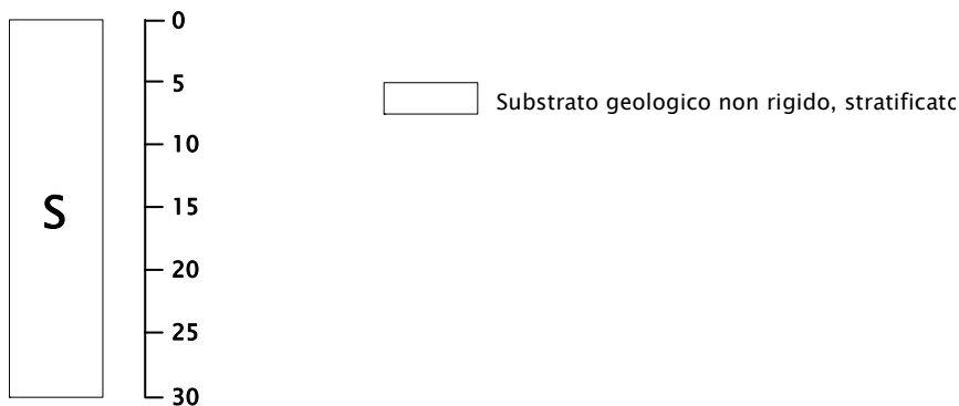
Figura 35 – Successione stratigrafica cod. 2001.
