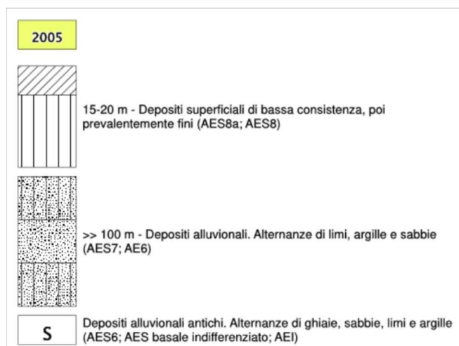
Figura 8.1 – Schemi dei rapporti stratigrafici rappresentativi della zona stabile
