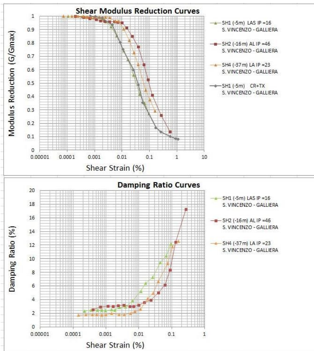
Figura 5.2 - Curve di decadimento dei sedimenti fini di San Vincenzo (sondaggio eseguito nella zona Campo Sportivo)
