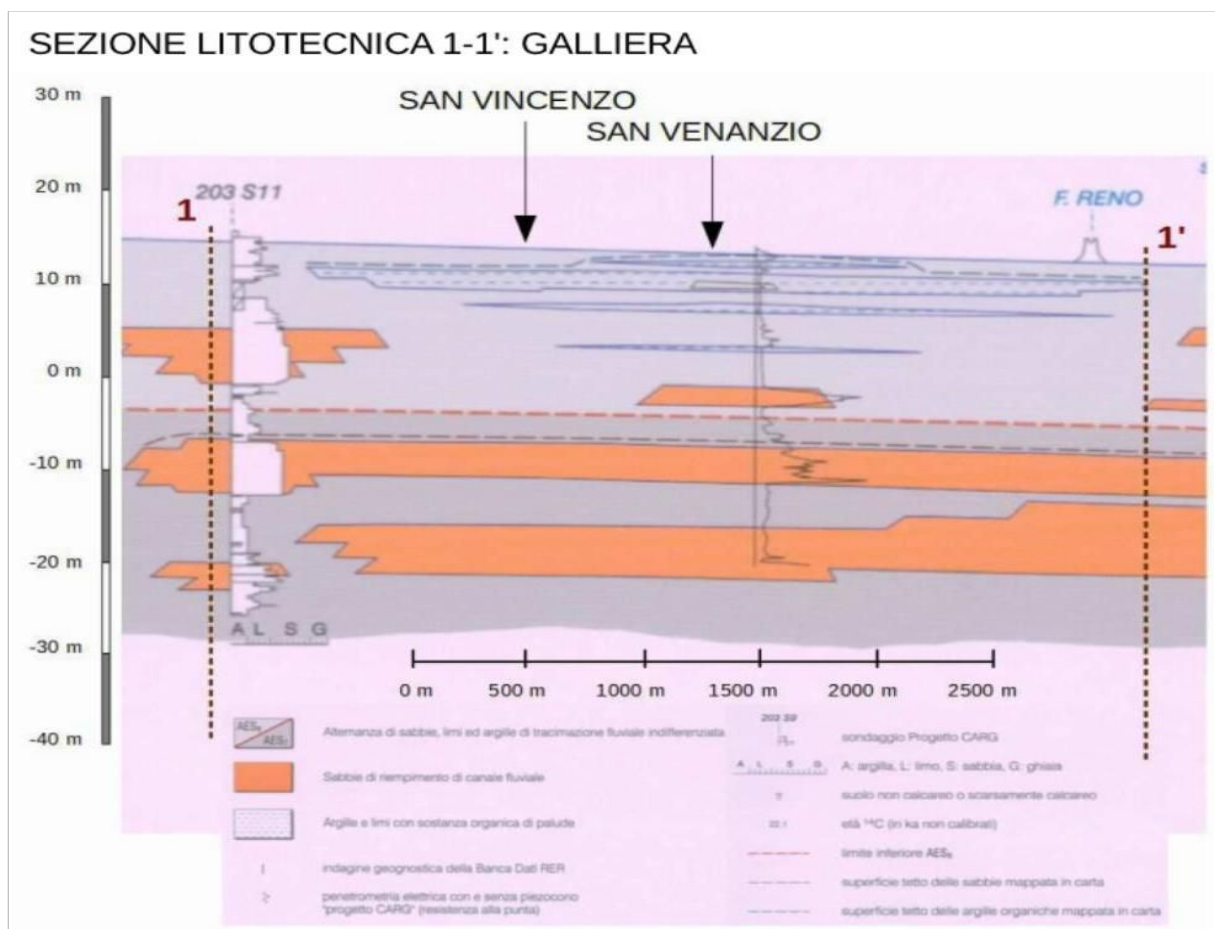
Figura 5.4 – Stralcio sezione litotecnica ISPRA (rinominata 1-1' per questo studio)
