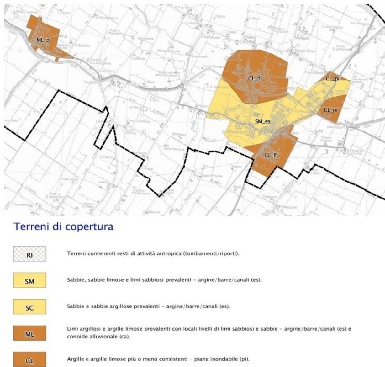
Figura 5.1 – Cartografia geotecnica di sintesi relativa al territorio comunale di Galliera
