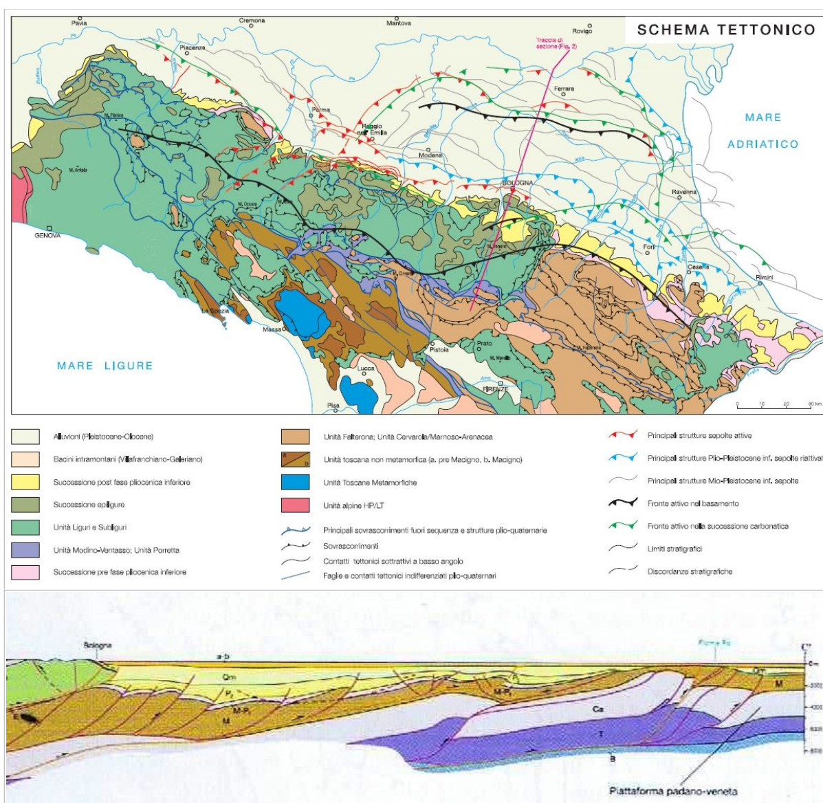
Figura 3.1 - Schema tettonico dell'Appennino Settentrionale - (Fonte: SGSS Regione Emilia-Romagna, 2004)
