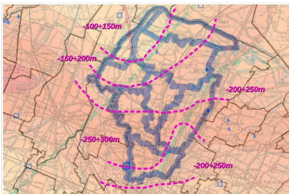
Figura 5.6 - Stralcio della Carta Sismotettonica della Regione Emilia-Romagna ed aree limitrofe (RER, 2016). Sono sovrapposti i confini comunali dell'Unione Reno e rimarcate le isobate della base del Sintema AES (m slm)
