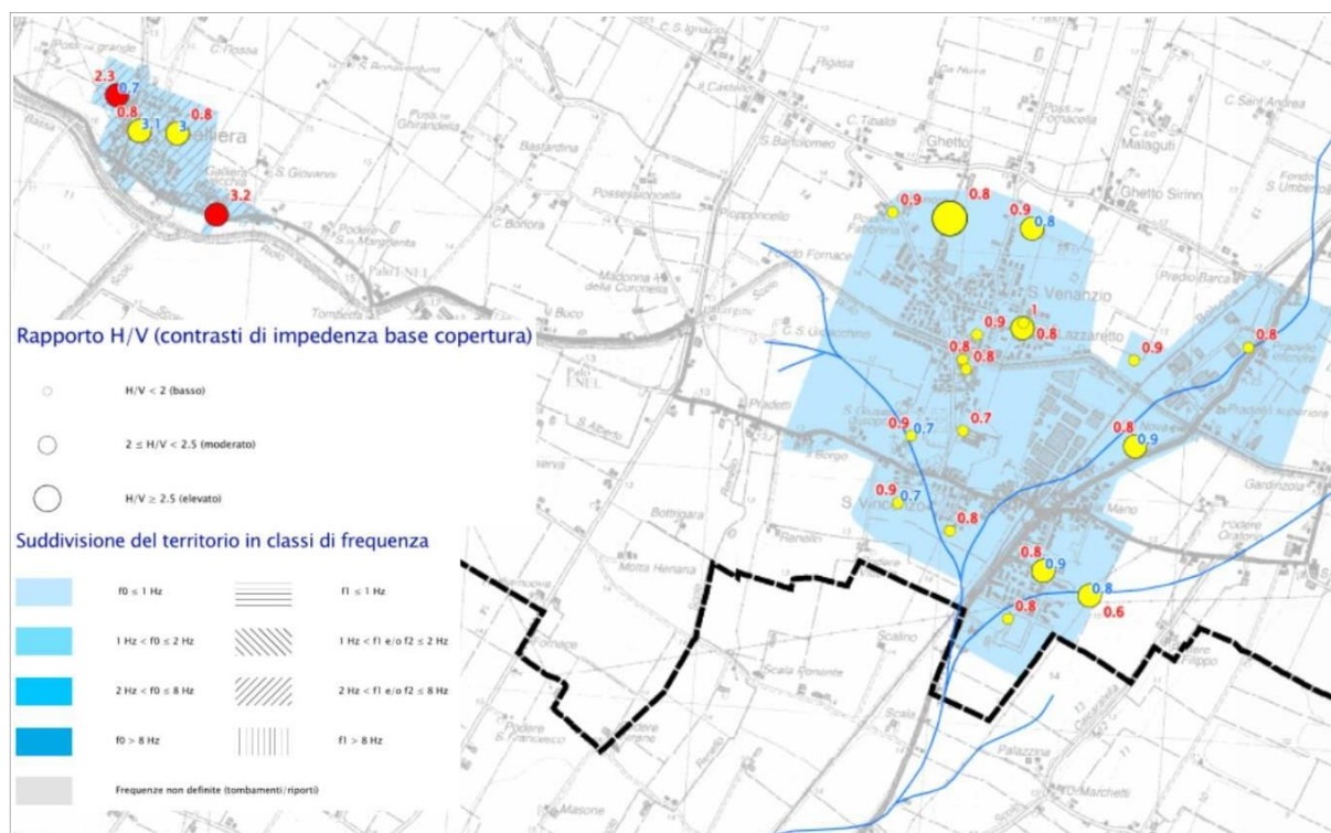
Figura 5.10 - Suddivisione del territorio urbano/urbanizzabile di Galliera in classi di frequenza naturale dei terreni. I colori rappresentano classi differenti. L'ampiezza dei cerchi classifica le massime amplificazioni spettrali ricavate dalle registrazioni HVSR
