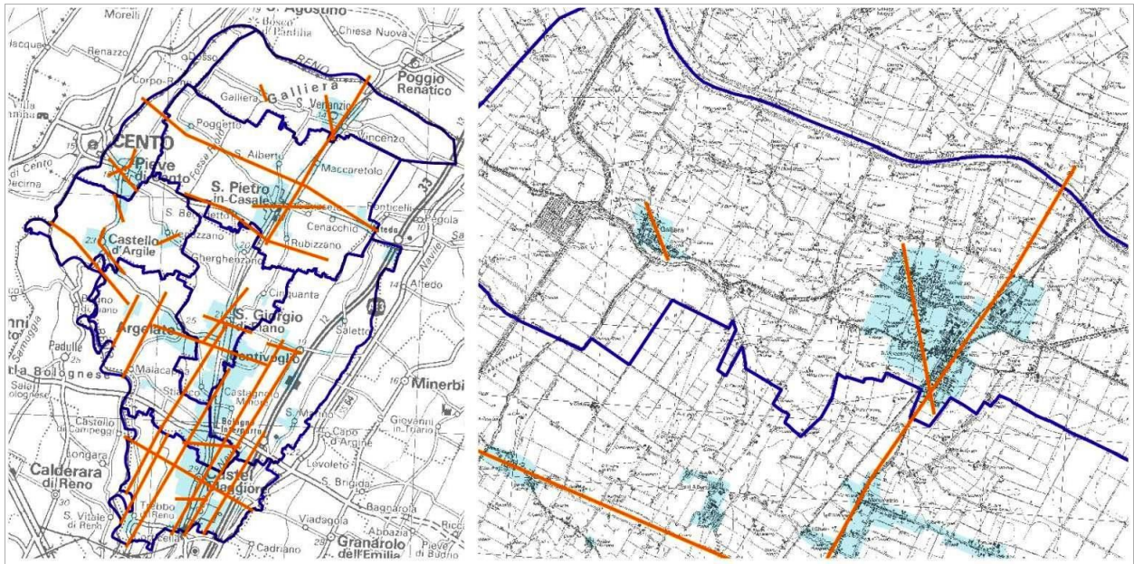
Figura 5.3 – Sezioni litotecniche di riferimento per lo studio di MS (Unione Reno Galliera e dettaglio di Galliera)
