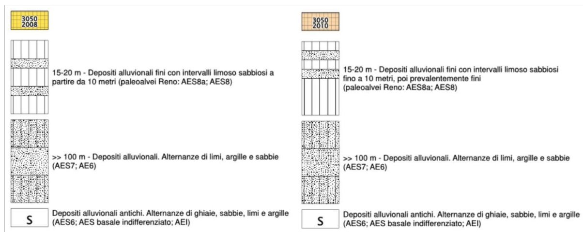
Figura 8.2 – Schemi dei rapporti stratigrafici rappresentativi delle zone di attenzione per instabilità
