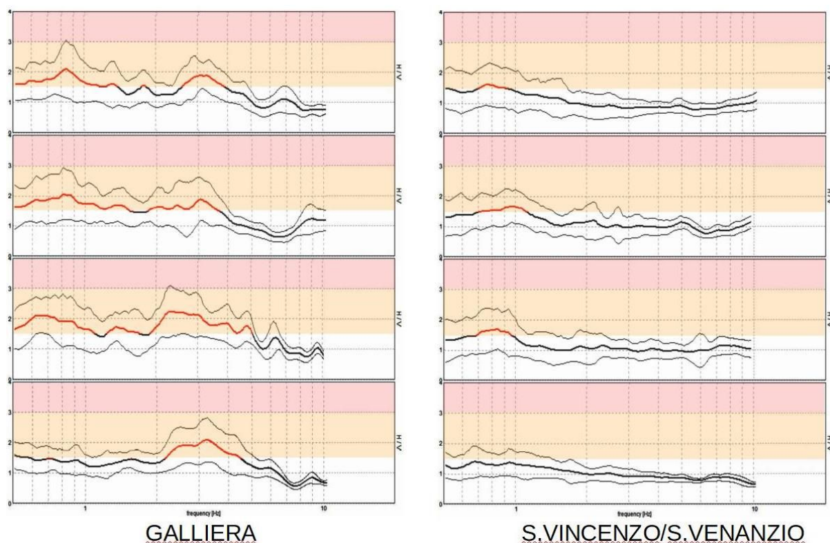
Figura 5.11 - Confronto tra spettri H/V ricavati da registrazioni HVSR nel Comune Galliera
