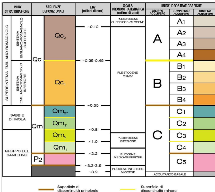
Figura 3.5 - Schema stratigrafico dei depositi plio - quaternari del bacino padano, con indicazione delle principali unità stratigrafiche, sequenze deposizionali e unità idrostratigrafiche (RER & ENI-AGIP, 1998)
