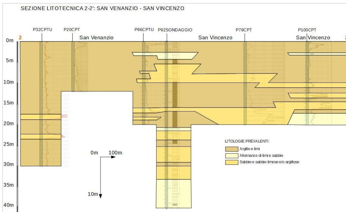
Figura 5.5- Sezione litotecnica 2-2' (San Venanzio - San Vincenzo) elaborata per questo studio
