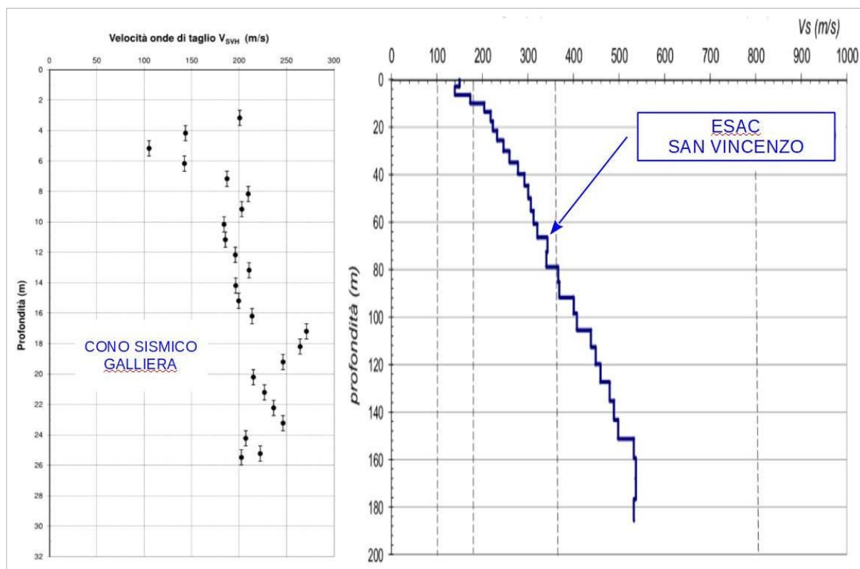
Figura 5.8- Sismostratigrafie ricavate dal “Cono Sismico” eseguito in località Galliera dallo stendimento ESAC eseguito a San Vincenzo
