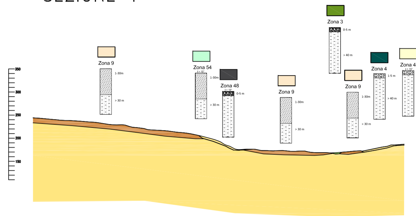
SEZIONE 3
