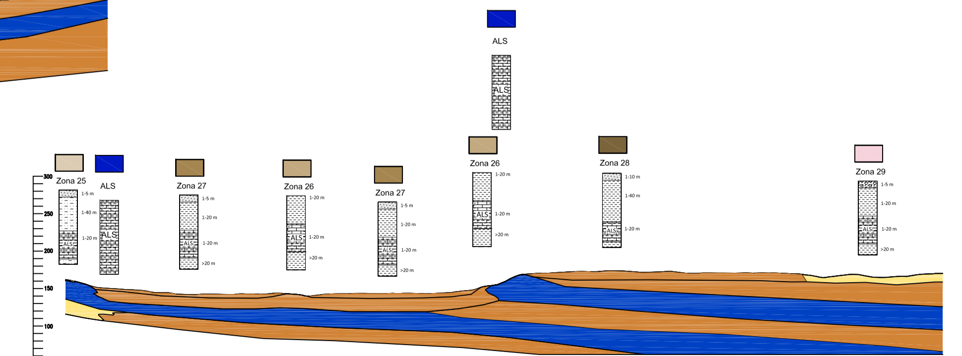
SEZIONE 9
