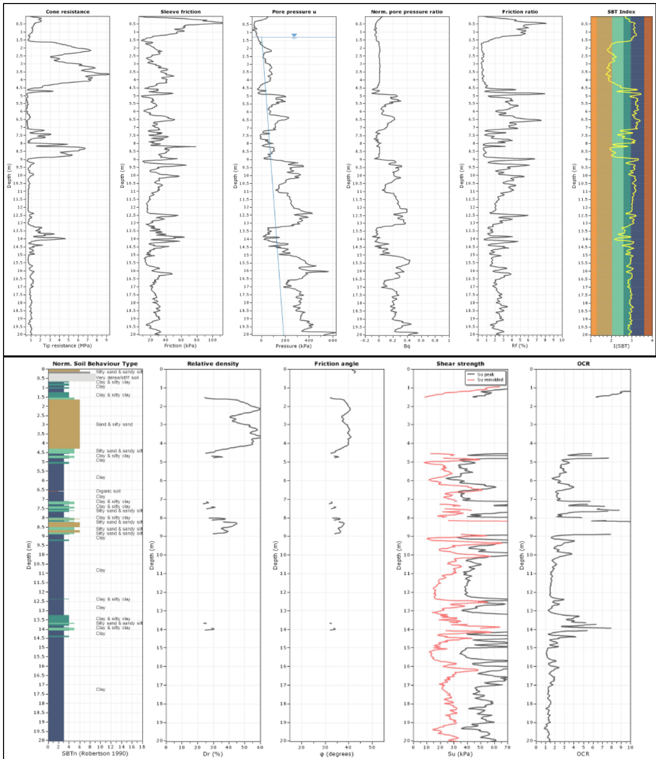
Figura 4.1-2 CPTU6 (Formignana Capoluogo)
