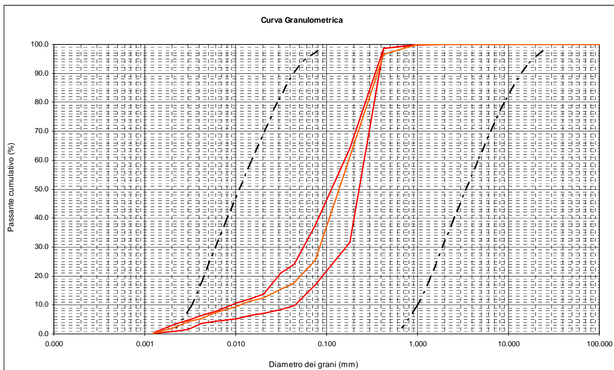
Figura 8.4.2-1 Confronto curva granulometrica dei campioni di sabbia prelevati a Formignana e fusi di riferimento normativi (coefficiente di uniformità U_c > 3.5 )
