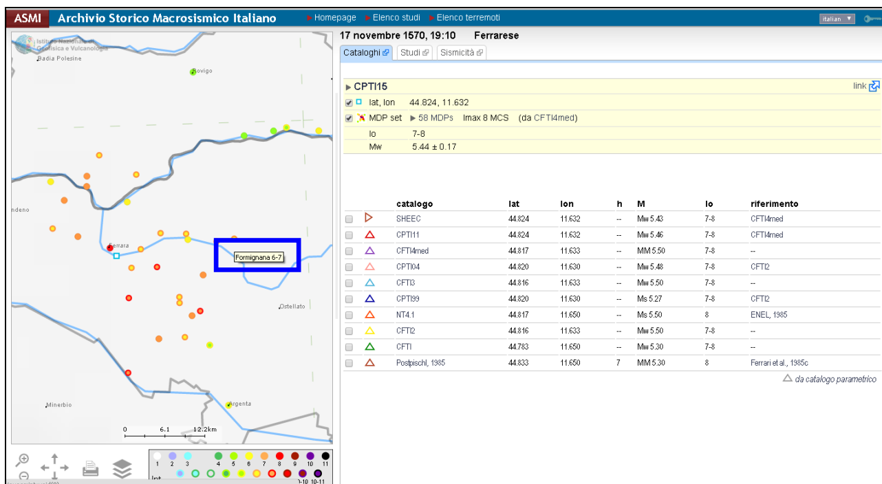
Figura 2.2-2: Localizzazione epicentro dell'evento principale che ha causato i maggiori effetti macrosismici sul comune di Formignana (FE) e valori di magnitudo associati. Nel riquadro l'area di interesse.
