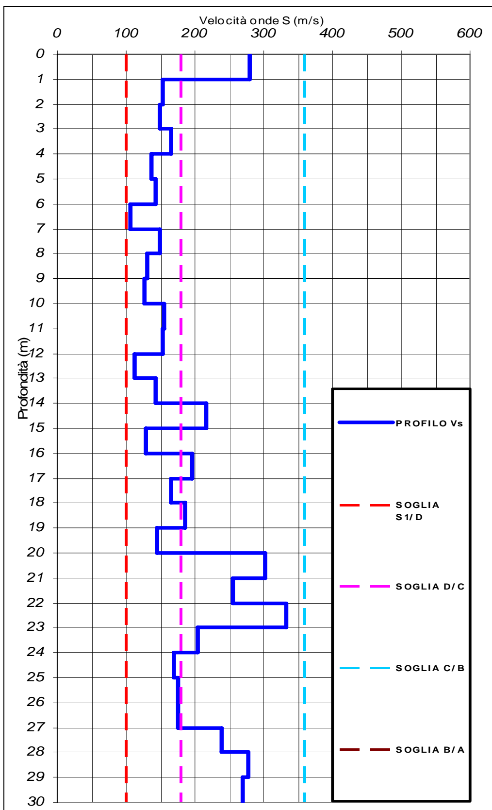
Figura 4.2-1 – Profilo di velocità onde S da SPTU4 eseguita presso Formignana capoluogo
