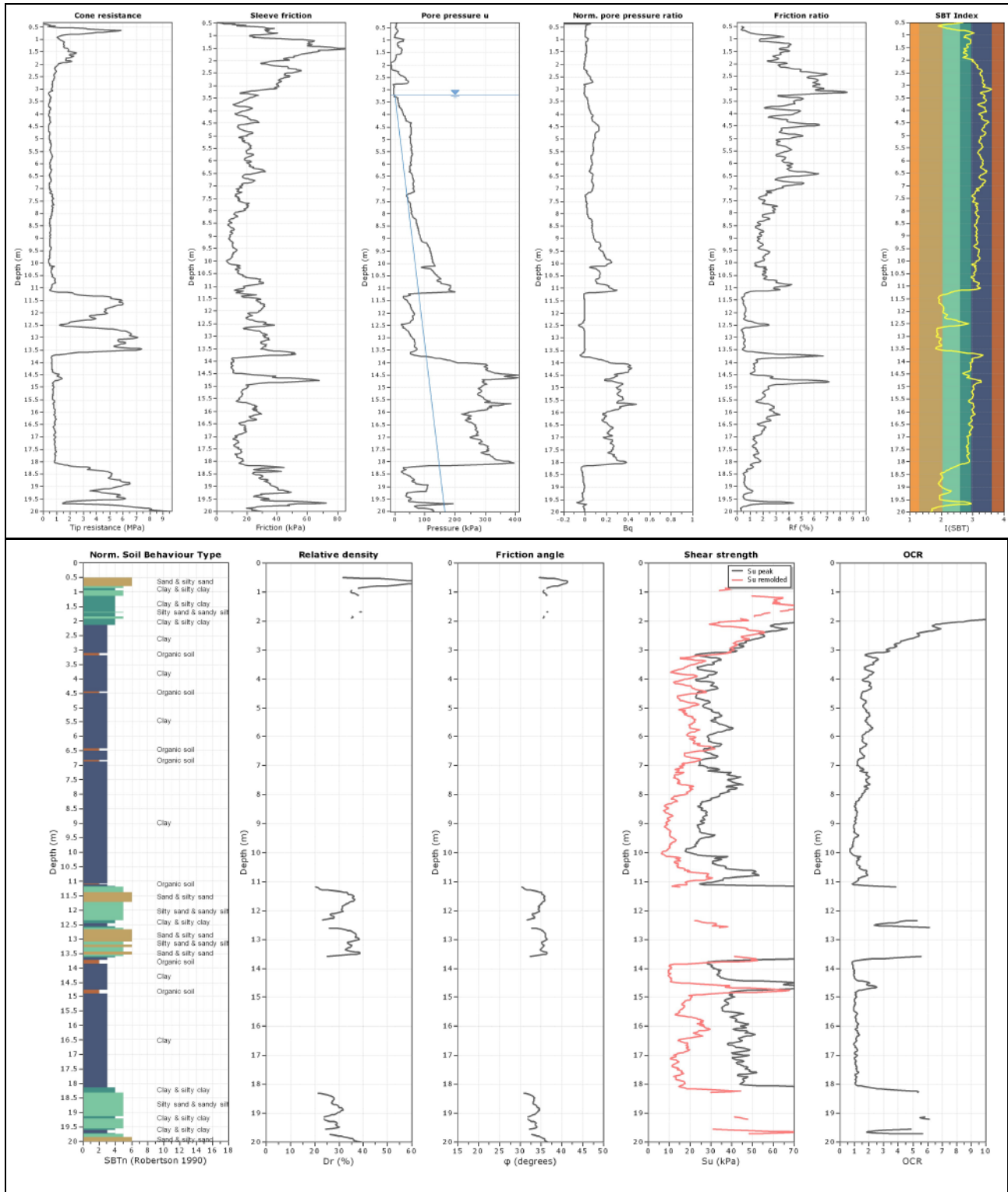
Figura 4.1-3 CPTU7 (Brazzolo Frazione)
