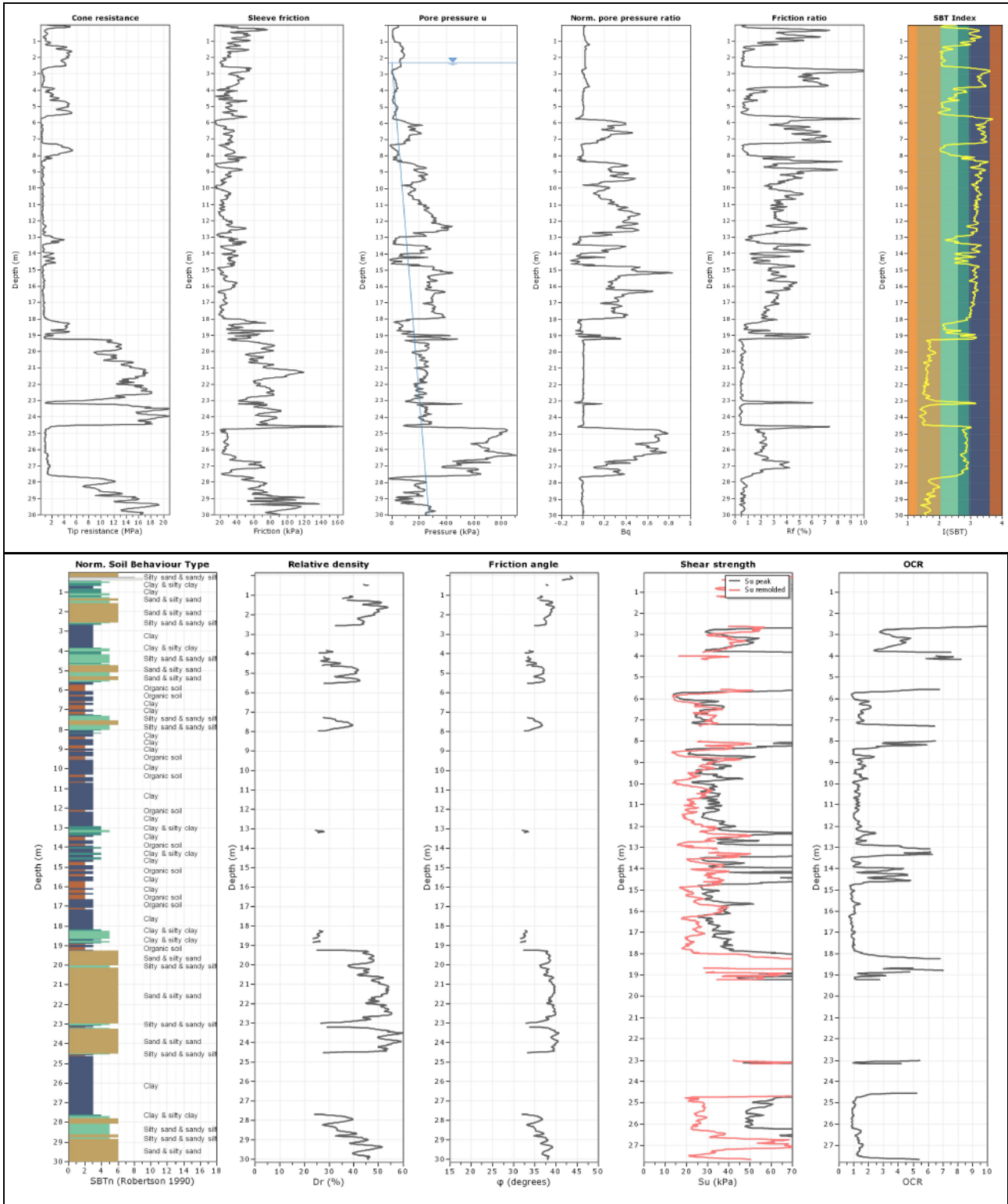
Figura 4.1-4 SCPTU4 (Formignana capoluogo)
