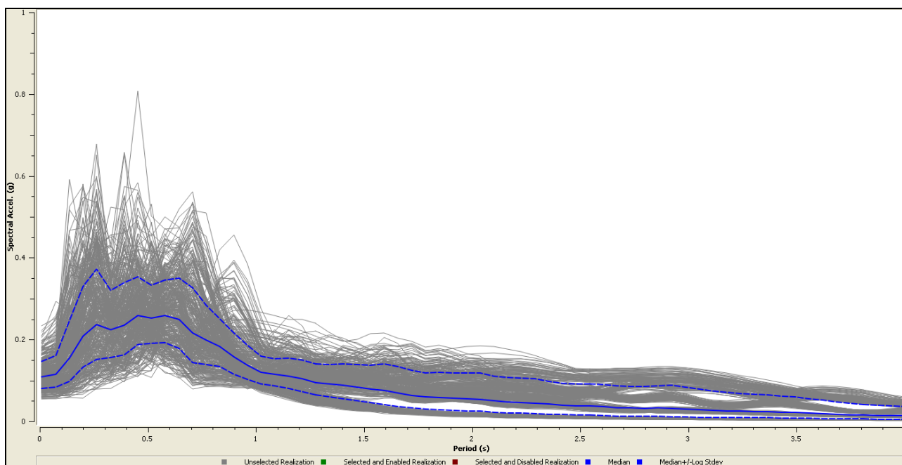
Figura 8.4.1-4 – Involuppo spettri finali calcolati per Formignana e frazioni
