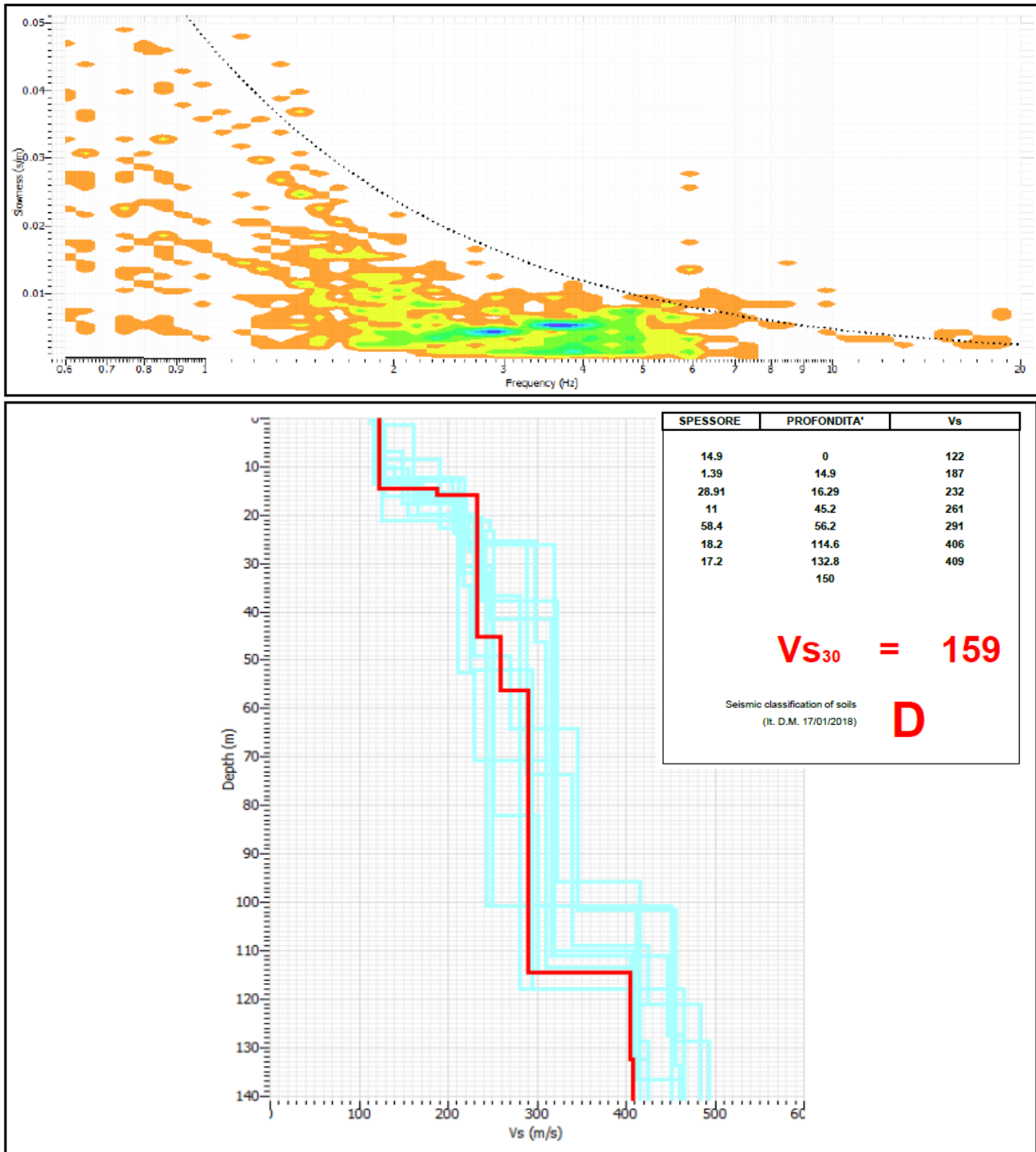
Figura 4.2-2 – ESAC (Formignana capoluogo)
