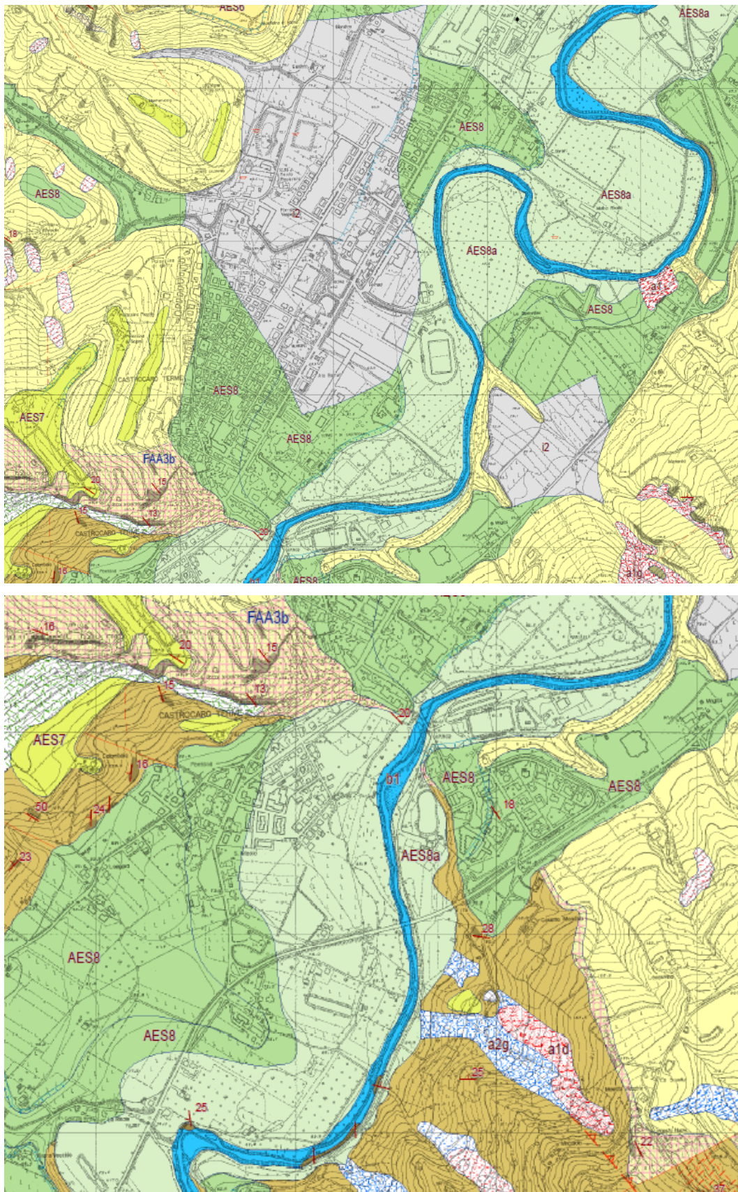
Stralcio della carta geologica regionale, elemento 254040 Castrocaro
