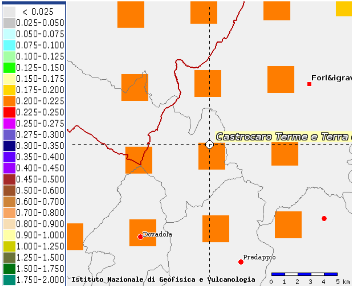
Figura 1 - MAPPA DI PERICOLOSITÀ SISMICA IN VALORI DI PGA con periodo di ritorno di 475 anni (pari alla probabilità di non eccedenza del 90% in 50 anni) Le aree a diverso PGA sono differenziate in base a colorazioni diverse corrispondenti alle diverse classi. (da ingv)
