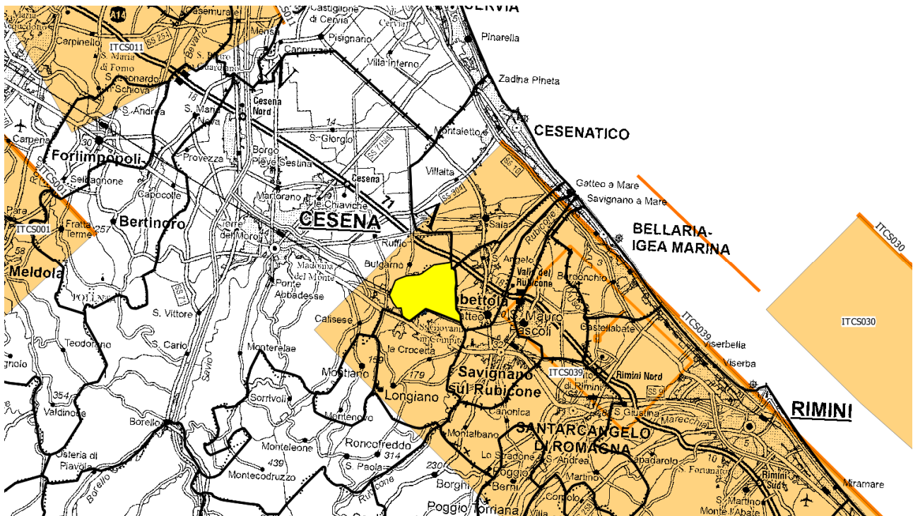
Figura – 3.4: Sorgenti sismogenetiche (Id-Nome-Max Magnitudo) individuate dal catalogo DISS 3.2.1 (Database of Individual Seismogenic Sources) dell’Istituto Nazionale di Geofisica e Vulcanologia.
