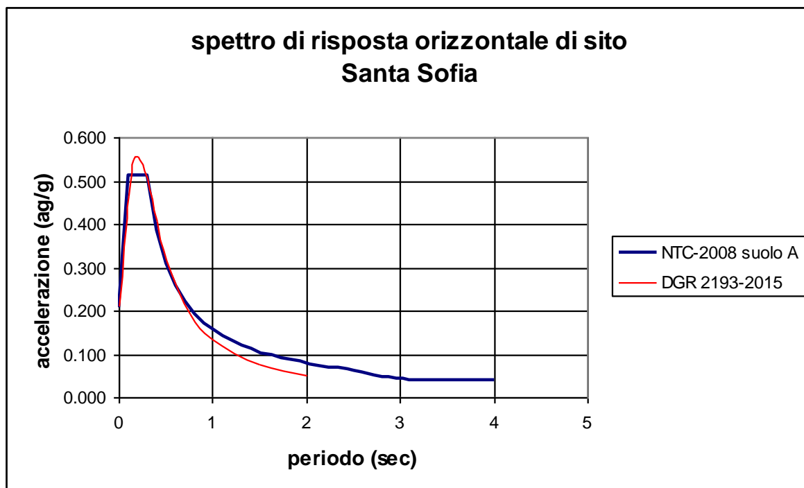
Figura n. 26 - Confronto tra spettro a probabilità uniforme e spettro di risposta elastico da NTC2008
