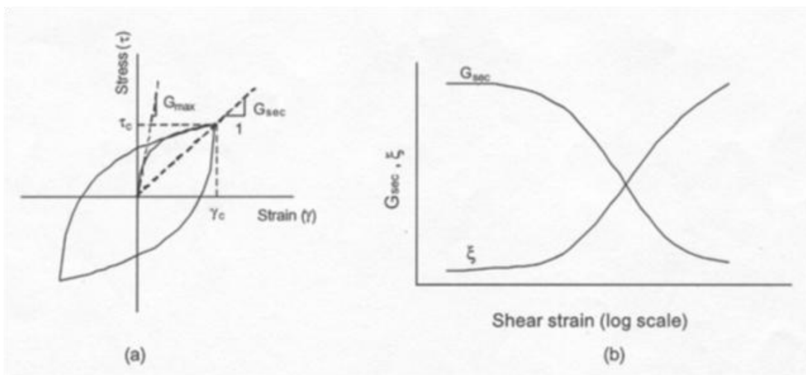
Figura n. 30 - Modello lineare equivalente: (a) curve tensioni - deformazioni; (b) variazione del modulo
