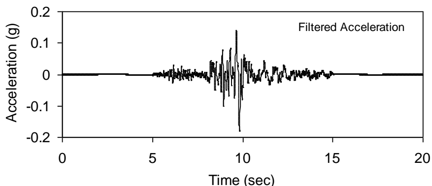
Figura n. 28b - Segnali di riferimento. Accelerogramma segnale 000126xa
