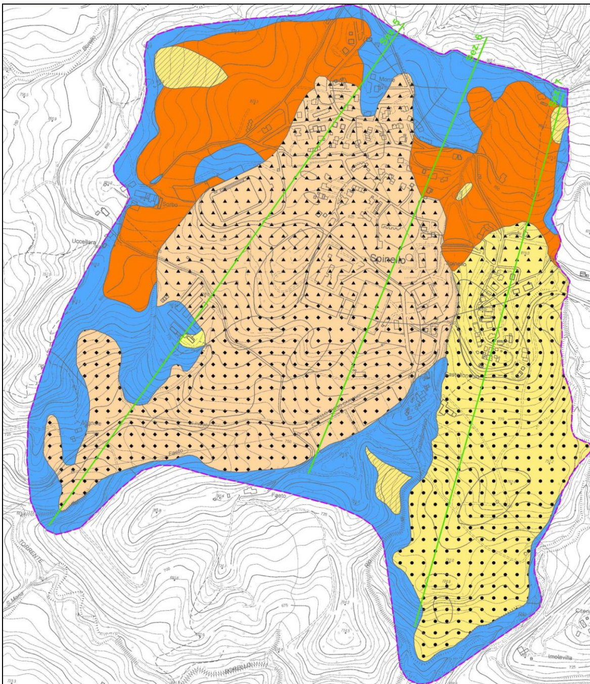
Figura n. 15 - Zona di Spinello interessata dagli approfondimenti di II e III livello
