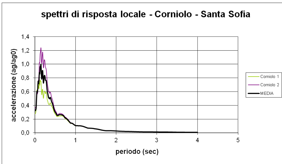
Figura n. 34 - Spettri di risposta sismica locale a Corniolo
