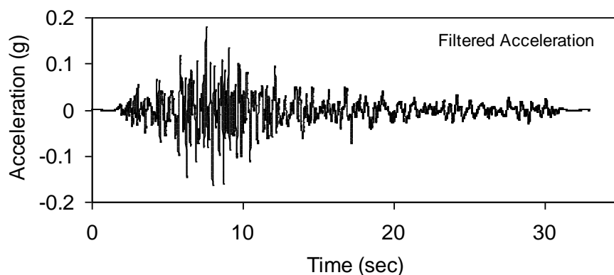
Figura n. 28c - Segnali di riferimento. Accelerogramma segnale 000354xa
