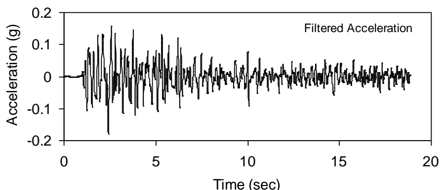
Figura n. 28a - Segnali di riferimento. Accelerogramma segnale 000046xa
