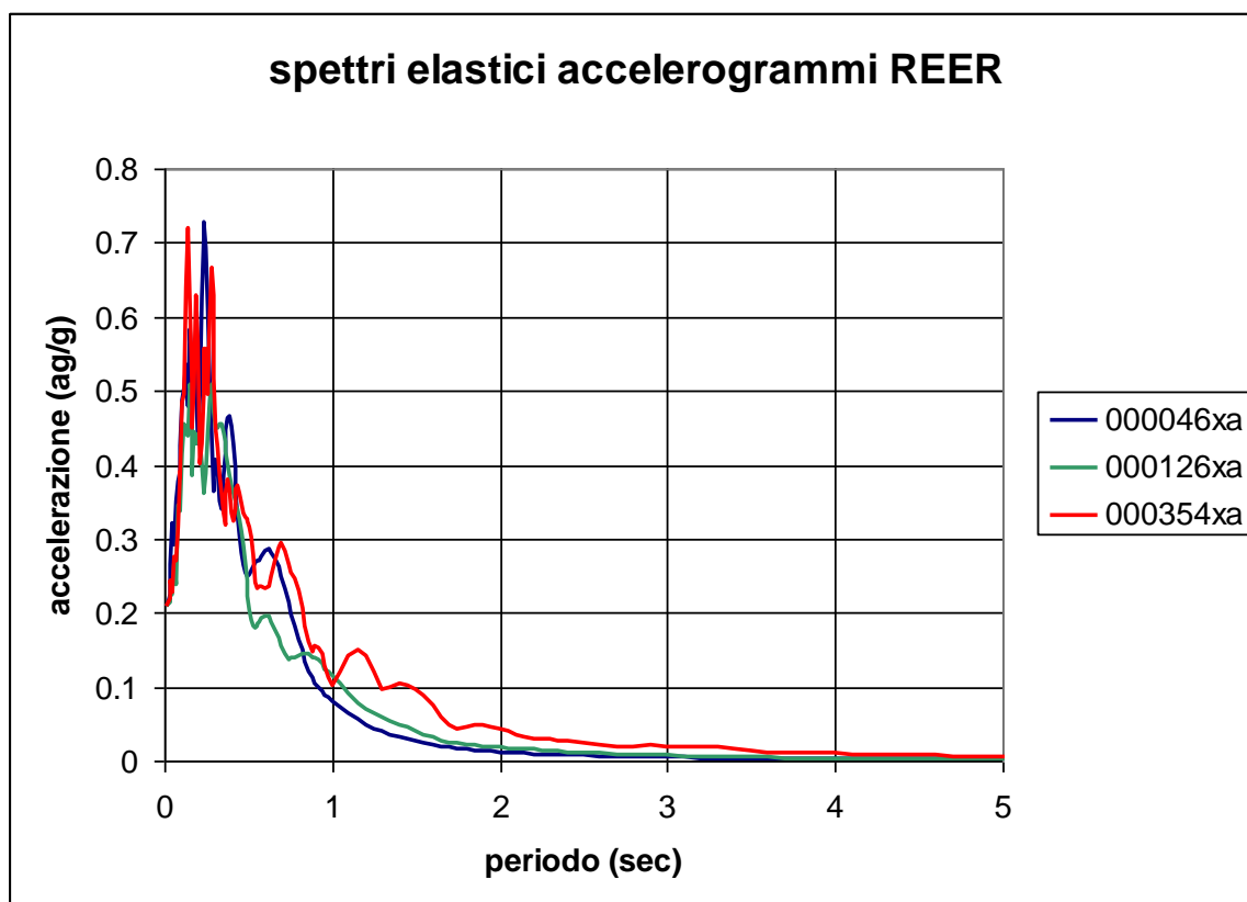
Figura n. 29 - Spettri dei segnali di input di riferimento
