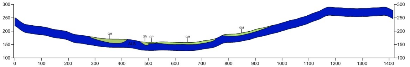
Sezione geologico-tecnica Modigliana
