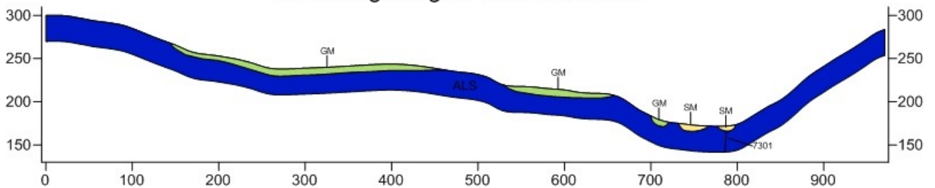
Sezione geologico-tecnica Sarsina
