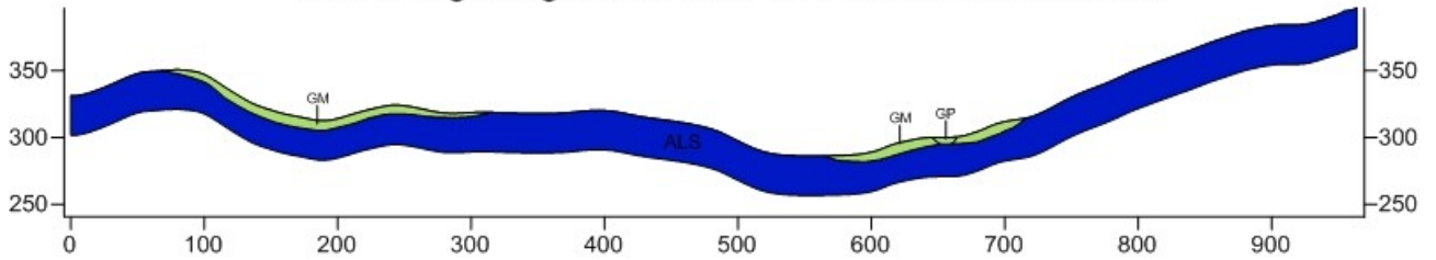
Sezione geologico-tecnica Portico e San Benedetto
