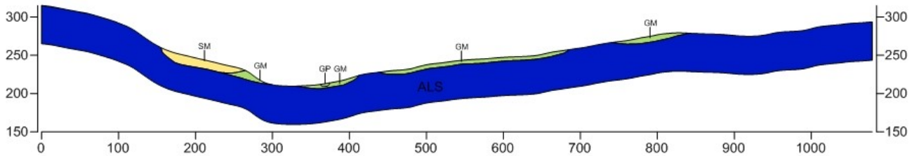
Sezione geologico-tecnica Rocca San Casciano
