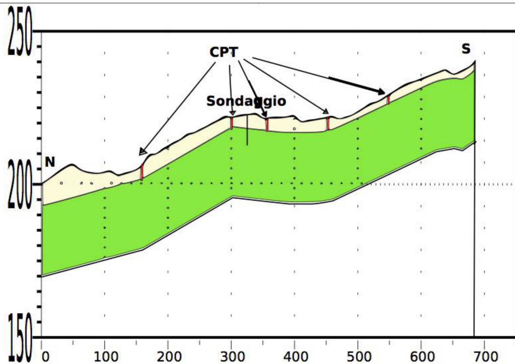
SEZIONE 1
