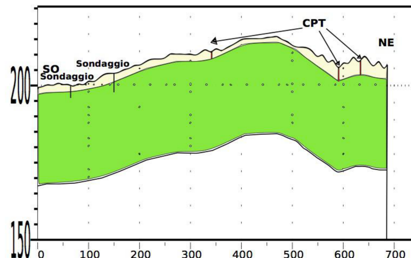
SEZIONE 2
